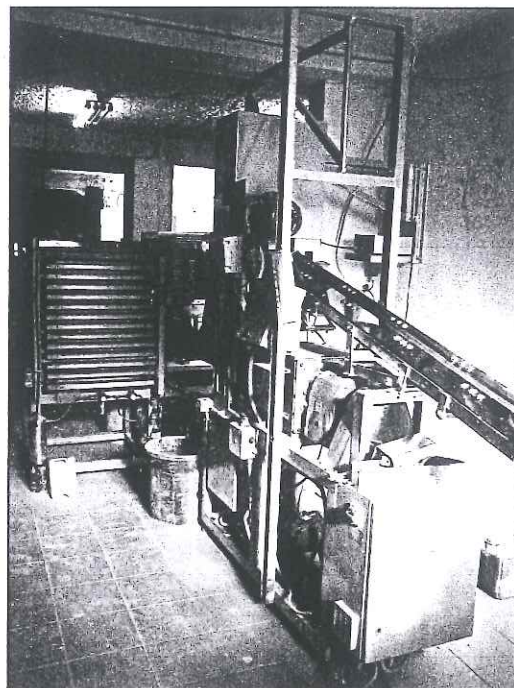
Univerzalna brizgalica BKP 300
